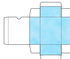
サック箱(キャラメル箱) ＜用途＞お菓子、石鹸、雑貨等に使われます。
